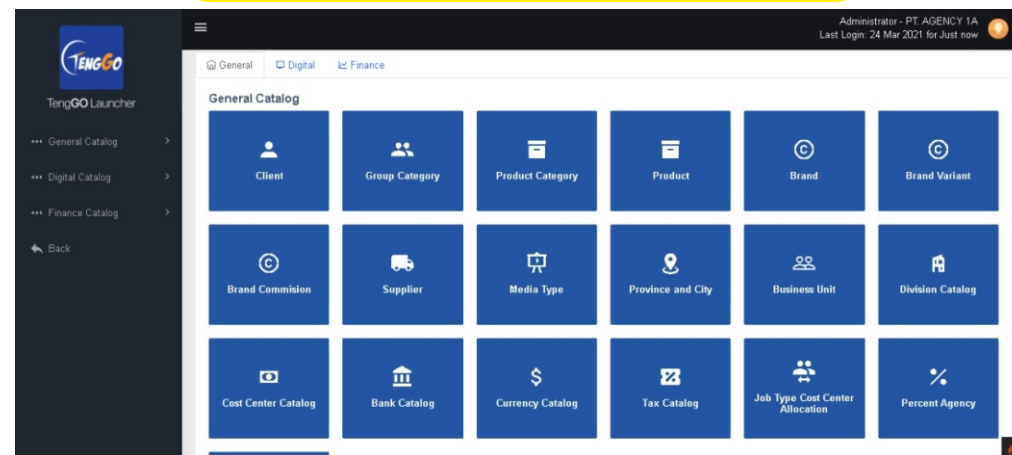
Web-app interface
