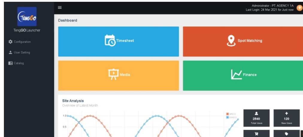
Web-app interface
