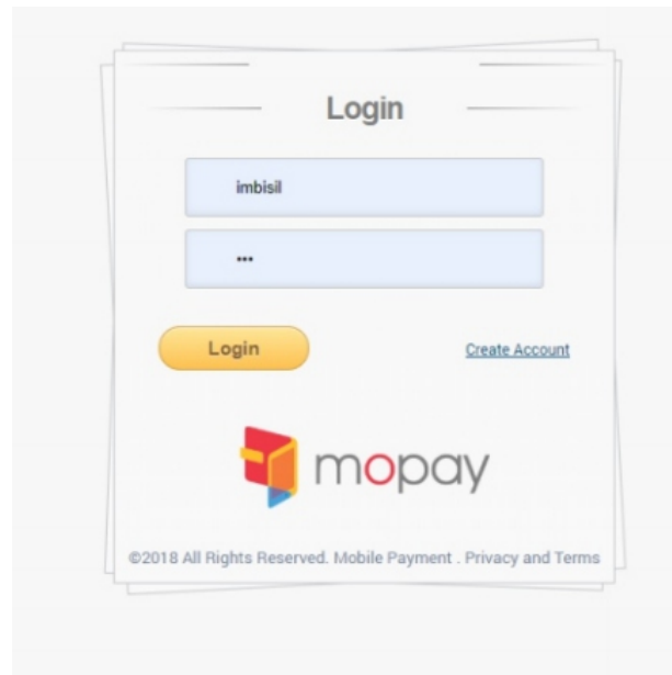
Login page
