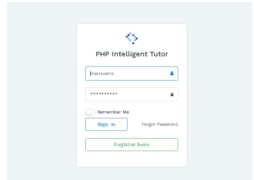
Login page
