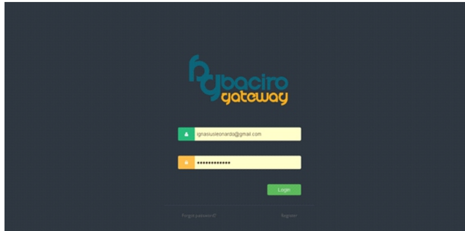
Login page
